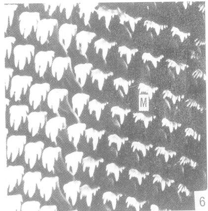
1. 折叠萝卜螺齿舌外形 \times 130 ; 2. 大脐圆扁螺齿舌带中部 \times 400 ; 3. 折叠萝卜螺齿舌, 示中央齿、侧齿 \times 1000 ; 4. 大脐圆扁螺齿舌, 示中央齿、侧齿 \times 2000 ; 5. 折叠萝卜螺齿舌, 示缘齿 \times 1000 ; 6. 大脐圆扁螺齿舌, 示缘齿 \times 2000 ; C: 中央齿 (central teeth); L: 侧齿 (lateral teeth); M: 缘齿 (marginal teeth)
